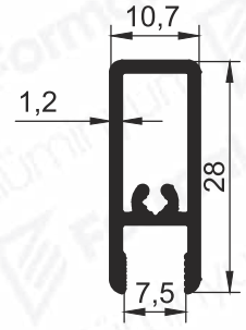
Pr.No: 9696 0,262 kg/m
