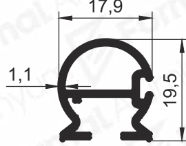
Pr.No: 9171 0,243 kg/m
