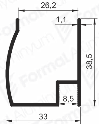
Pr.No: 9755 0,342 kg/m
